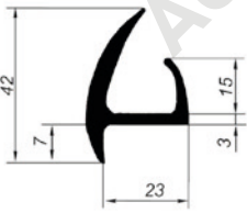
Уплотнитель ворот резиновый (23мм, 2,6м) 829382
