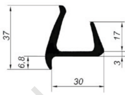
Уплотнитель ворот резиновый (30мм, 2,6м) 815615
