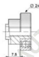
Ролик низкий под заклепку с юбкой 7,5 мм сдвижной крыши
