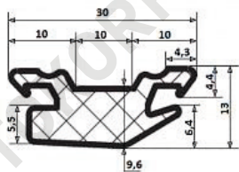
Профиль уплотнительный для контейнера Ширина (мм): 30 841785
