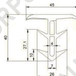
Профиль уплотнительный между контейнерами длина – 12 м/п 841840
