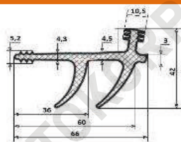
Профиль уплотнительный для контейнера Ширина (мм): 66 841786
