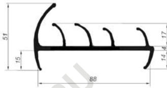
Уплотнитель ворот для рефрижератора 4-х лепестковый 815298
