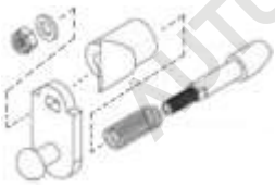
Фиксатор сдвижной крыши Krome EDSCHA
