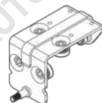
Каретка роликовая (5 роликов) EDSCHA 789710
