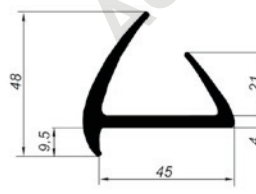
Уплотнитель ворот резиновый (45мм, 2,6м) 815868
