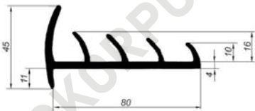
Уплотнитель ворот резиновый 4х-лепестковый (80мм, 2,6м) 823181
