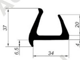
Уплотнитель ворот резиновый (34мм, 2,6м) 815865
