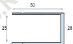
Окантовочный профиль 815705
