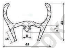
Профиль уплотнительный для контейнера Ширина (мм): 49 815867
