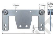
Ролик стойки
