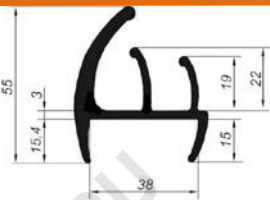
Уплотнитель ворот для изотермического фургона 815869
