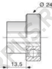
Ролик под болт с юбкой 13,5 мм сдвижной крыши
