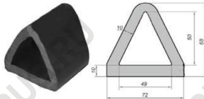
Буфер (отбойник) резиновый 2500x72x68 мм
