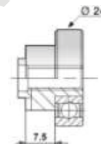
Ролик 24 мм под болт с юбкой 7.5 мм
