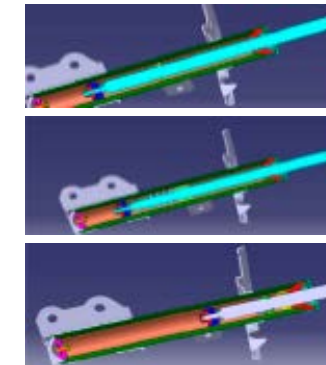
Моделирование конструкции буферизации для конструкции модуля пневматической рессоры
