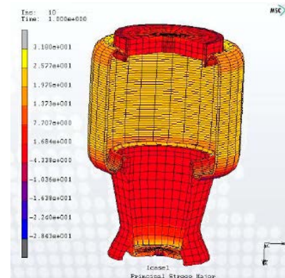
Моделирование конструкции пневматической рессоры
