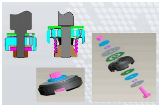
Многоклапанная система
