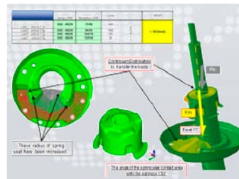
Симуляция CAE
