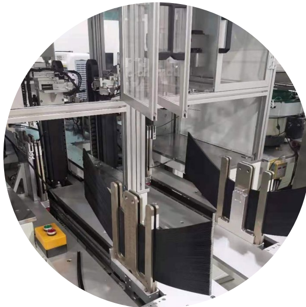
Автоматическая линия сборки бескаркасных щеток стеклоочистителя
