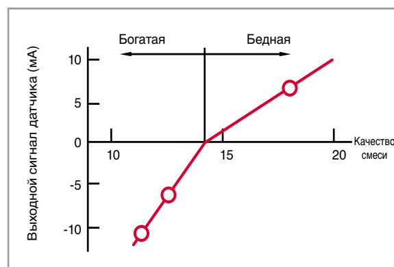
Рис. 7: Выходной сигнал датчика воздух/топливо
