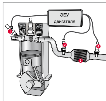
Рис. 1: Двигатель с каталитическим нейтрализатором и датчиками
