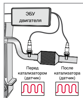
Рис. 5: Выходной сигнал при неисправном нейтрализаторе
